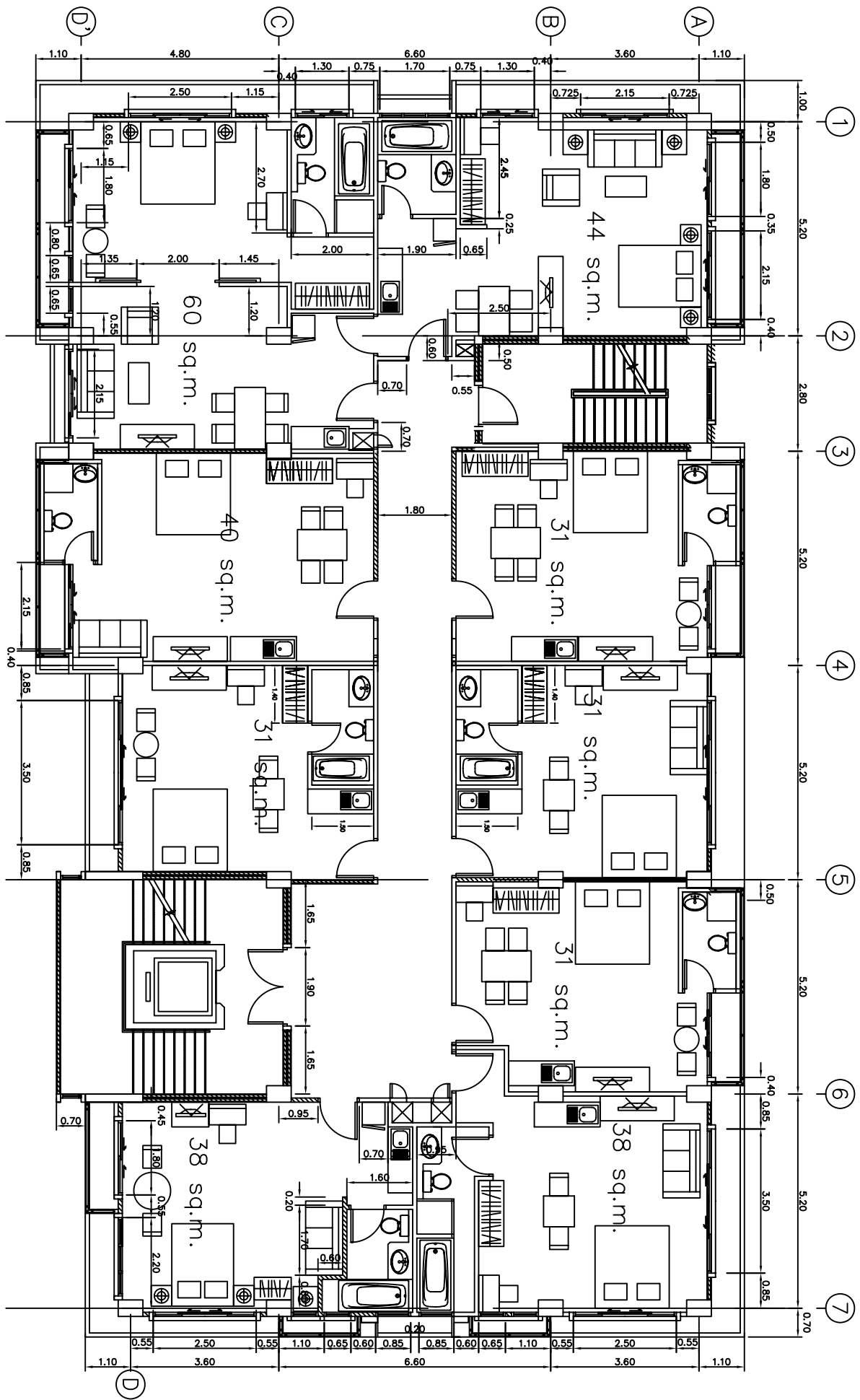
የአካላዊ ግንባታ ስራ ስራ ሰነድ 3 KEY PLAN
